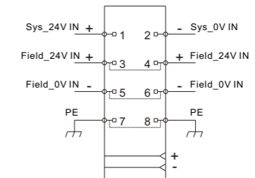
DF20-C-PN-RT-V1
