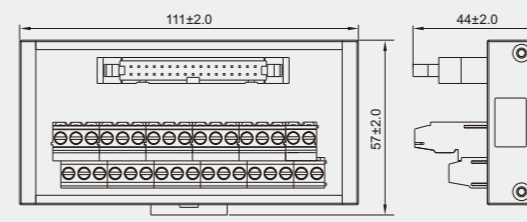
DM50-IDC-34-34-4Y-00A(H)
