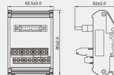
DM72-IDC-20-20-4Y-00A(H)
