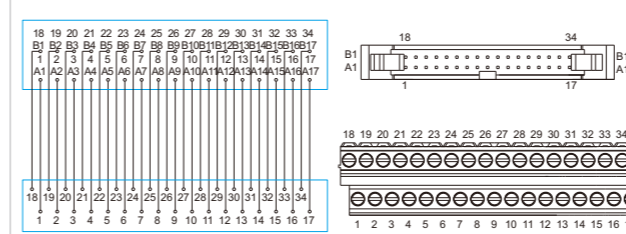
DM72-IDC-34-34-4Y-00A(H) DM50-IDC-34-34-4Y-00A(H)
