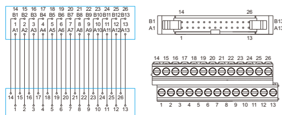
DM72-IDC-26-26-4Y-00A(H) DM50-IDC-26-26-4Y-00A(H)
