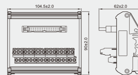
DM72-IDC-34-34-4Y-00A(H)
